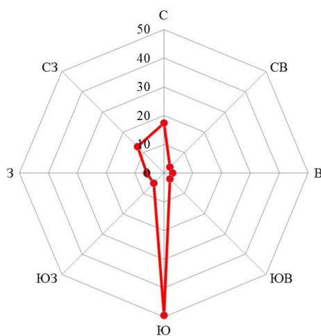
Рисунок 3.3.2 – Роза ветров за июль по данным метеостанции Юрты
