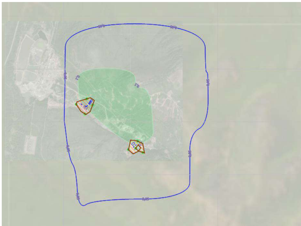
Рисунок 4.2.1 – Зона влияния 0,05 ПДК без учета действующих источников предприятия
